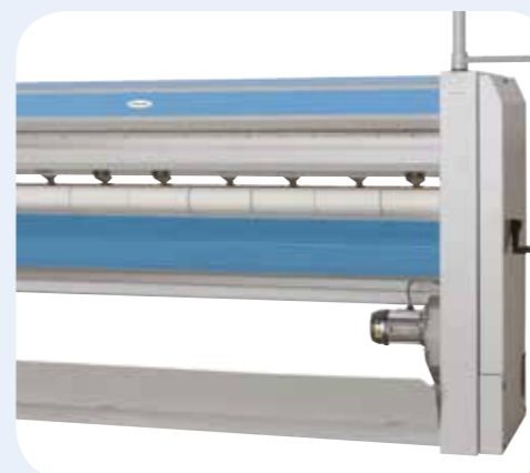
MANGANI ESSICCANTI Piano di stiratura 1625 mm. / 2065 mm. rullo Ø 325 mm. Dimensioni LxPxH: 2030x690x1645 mm. Dimensioni LxPxH: 2445x690x1145 mm.
